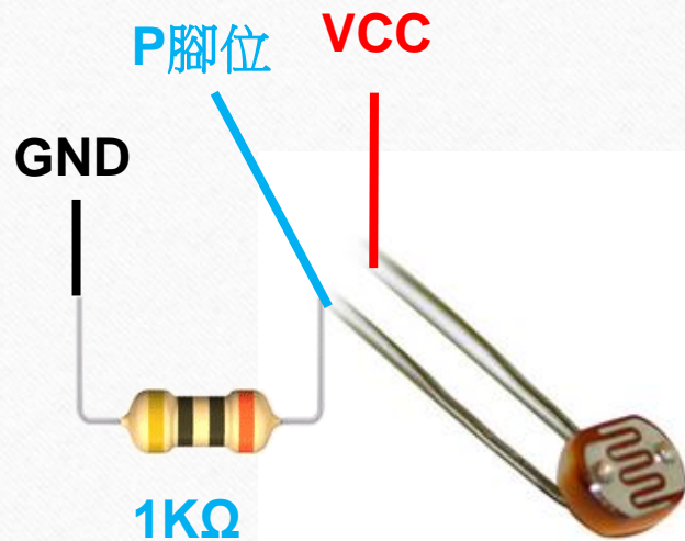
光敏電阻
