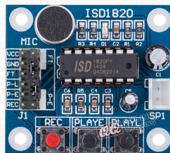
ISD1820簡易錄放音模組
