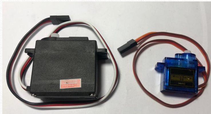
DS04-NFC 360°舵機
